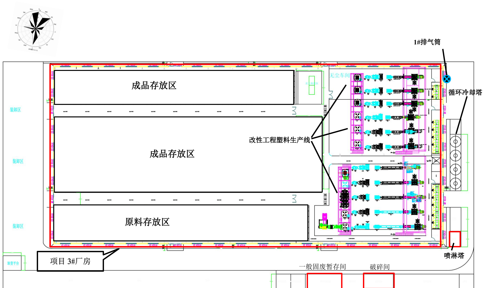
附图 2-2 3#厂房总平面布置示意图
