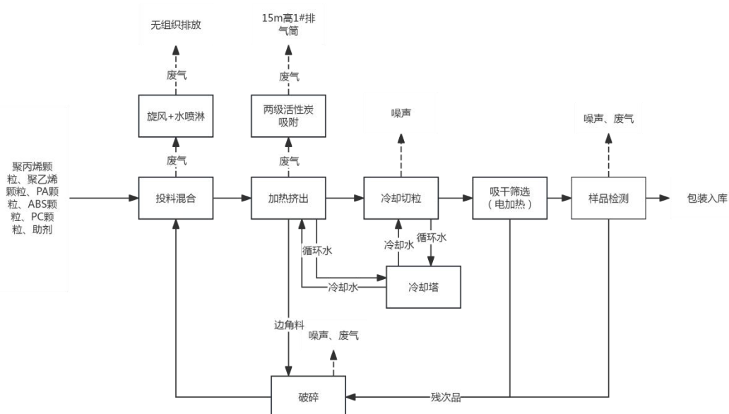
图 1 改性工程塑料生产工艺流程及产污节点图
