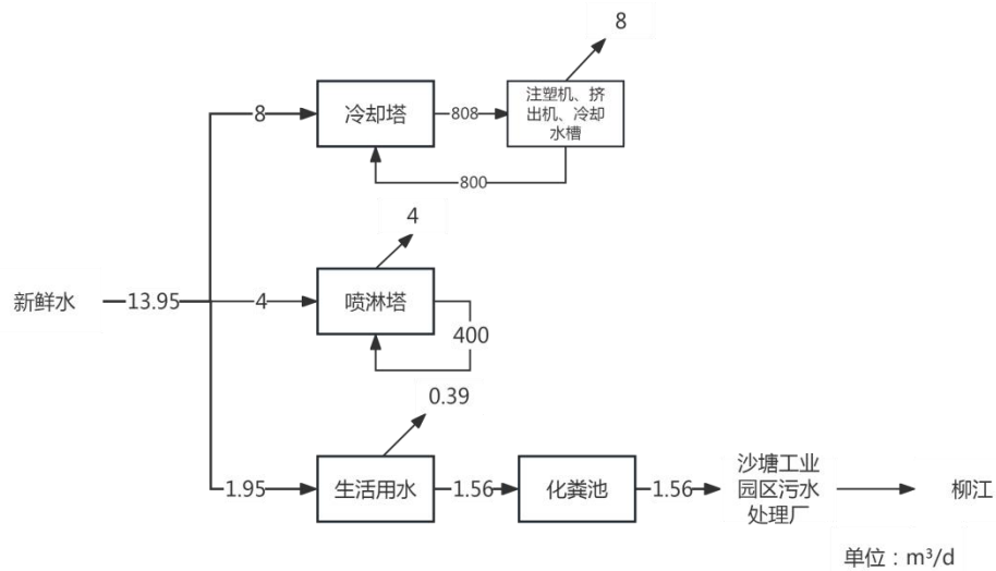
图 1 项目水平衡图
